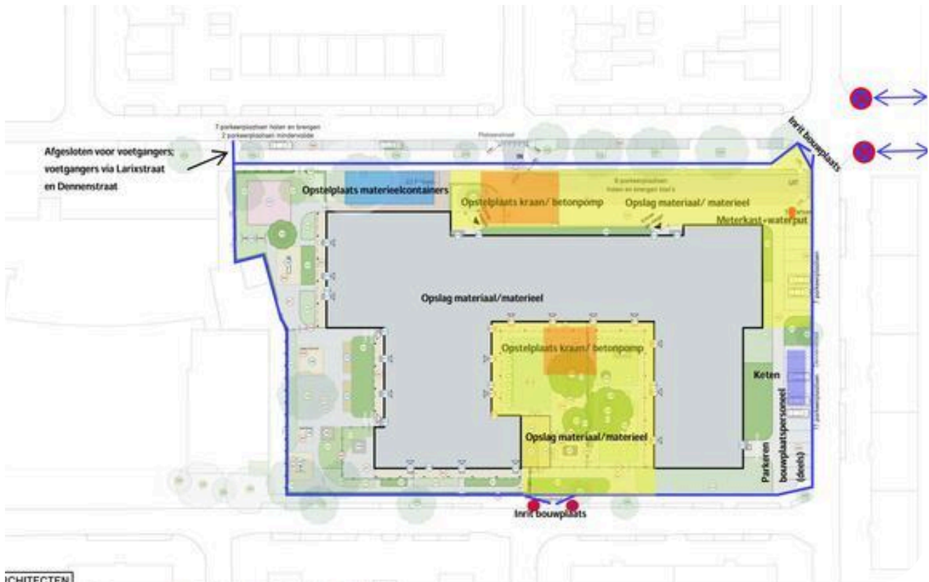
Afbeelding 3: Inrichting bouwplaats
